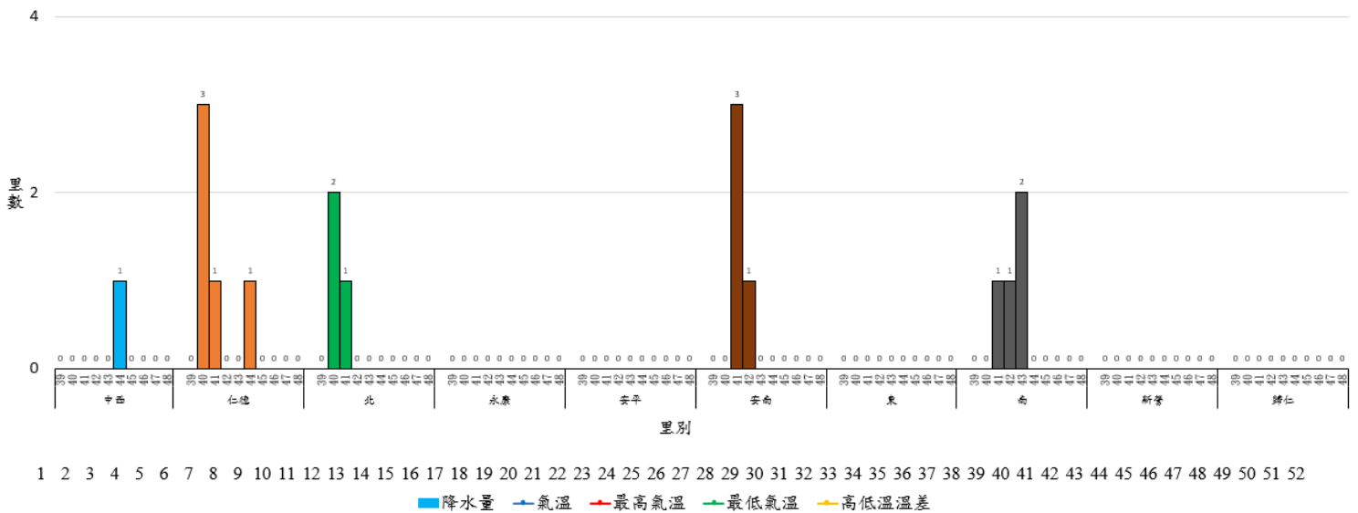
114年第39週至114年第48週臺南市監測區誘卵桶監測陽性率高於60%各區里數比較圖
